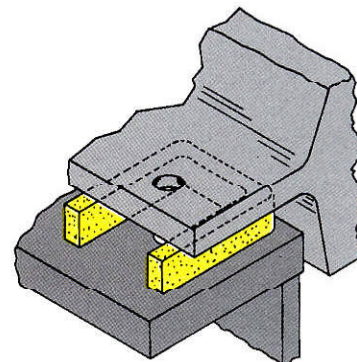
Fig. 2: Insert Damming per Chocking Plan
